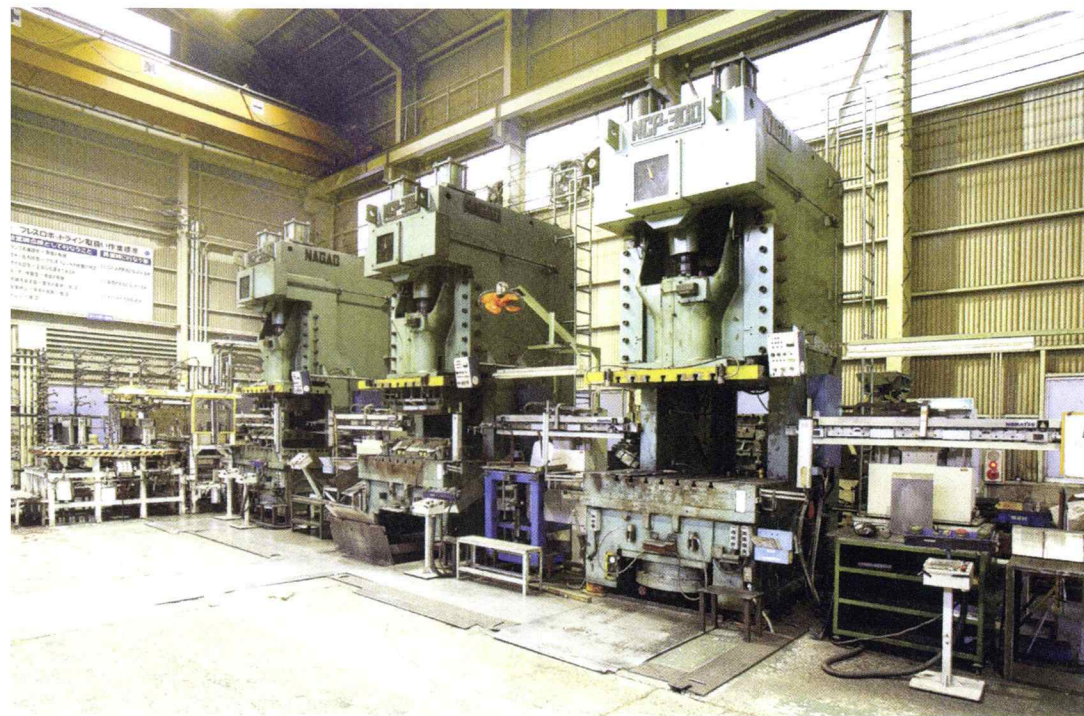
プレスロボットライン
