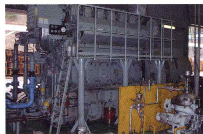
自家発電機
