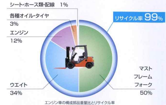
エンジン車の構成部品重量比とリサイクル率
