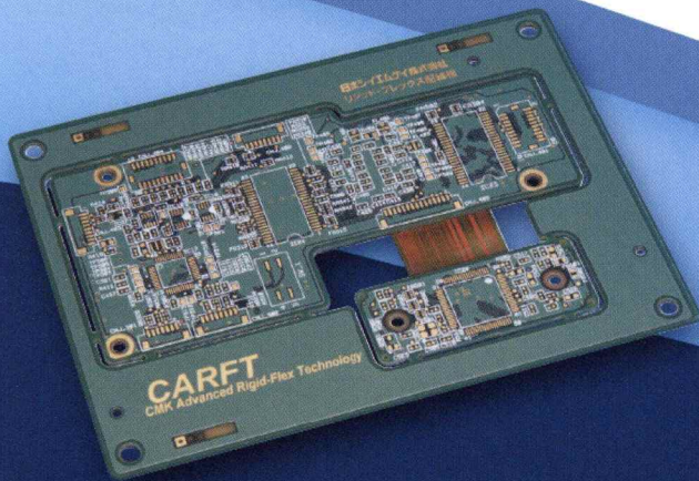
自動車用リジッドフレックス基板の『CARFT®』 高い信頼性で自動車ニーズに応えます
