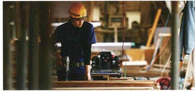
02. 図面から、出来上がりの形をイメージし、必要な型枠・材料を拾い出します
