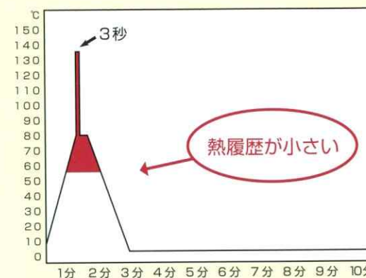
【スチームインジェクションの温度履歴】
