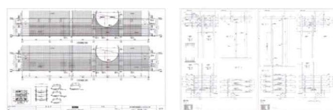
土木(配筋図)
