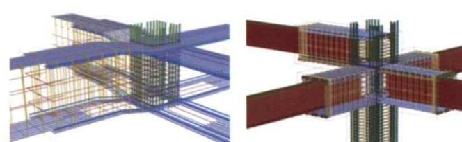
3D 納まり図
