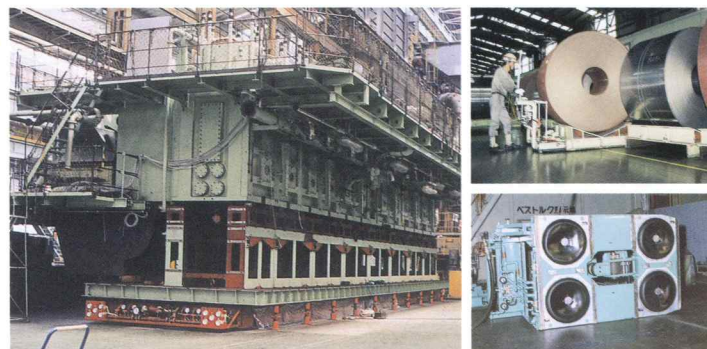
重量物搬送装置「AIR BEARING」
