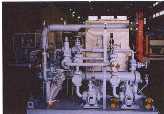
ミル減速機用潤滑油装置
