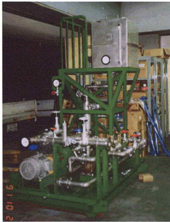
冷却水ユニット(CCWユニット)
